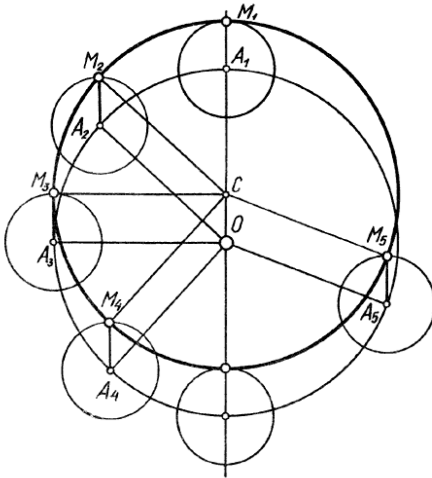
Рис. 3. Изображение перемещений «верхней» планеты с помощью движений по эксцентру и эпициклу. Планета M обращается вокруг Солнца C по окружности, которая по отношению к Земле O является эксцентром. То же движение можно представить в виде движения планеты M по эпициклу с центром A , который обращается по окружности с центром O (деференту)
